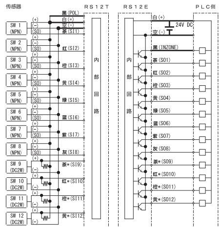
■ OXR-RS12系列配线图 (NPN规格)
