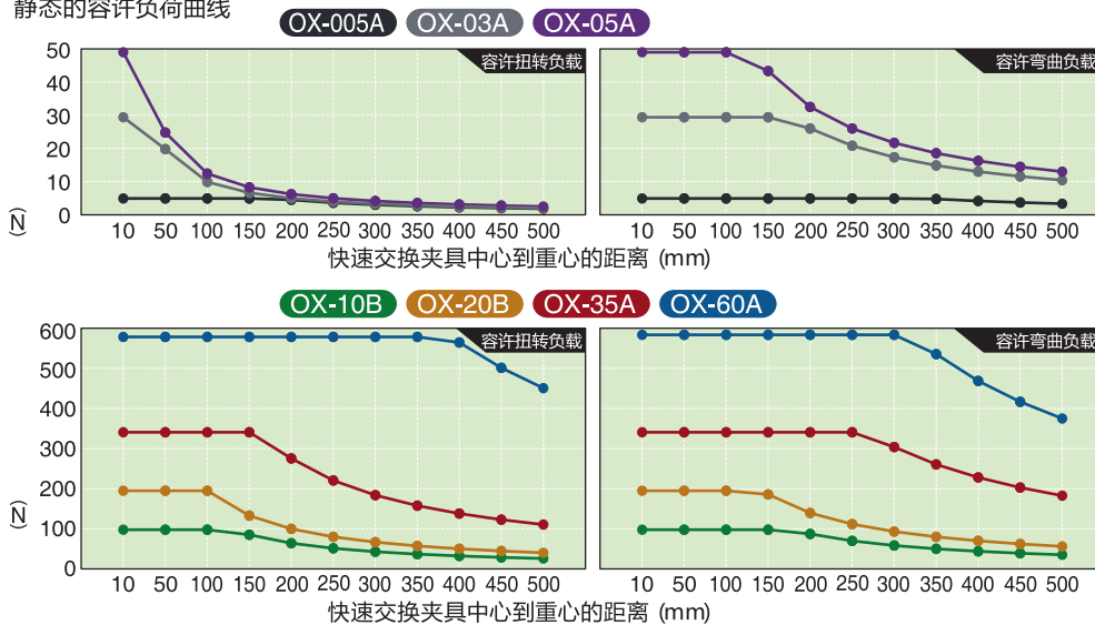
静态的容许负荷曲线
