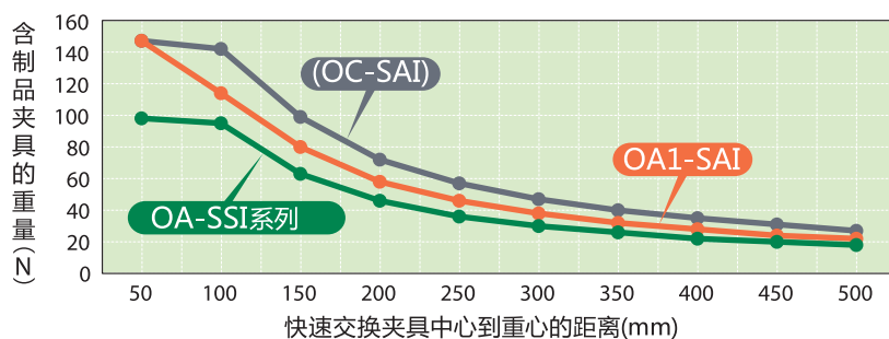
OA-SSI,OA1-SAI(OC-SAI)的静态的许容负荷曲线 (OA-LAI、OC-LAII的比较在 1-4)
