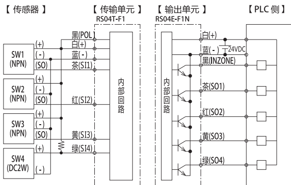
■ OXR-RS04系列配线图 (NPN规格)
