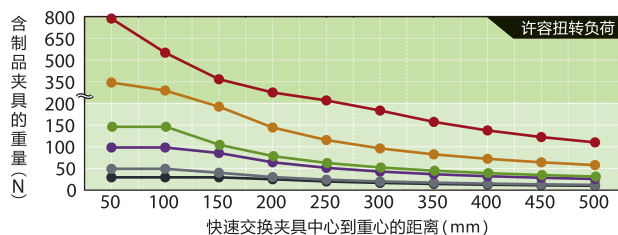
OX-A系列各静态的许容负荷曲线
